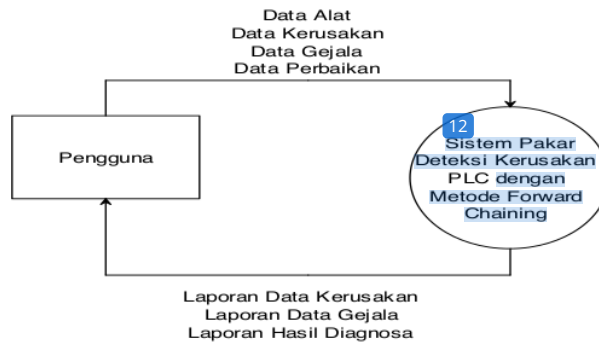
Gambar 1. Diagram Konteks
