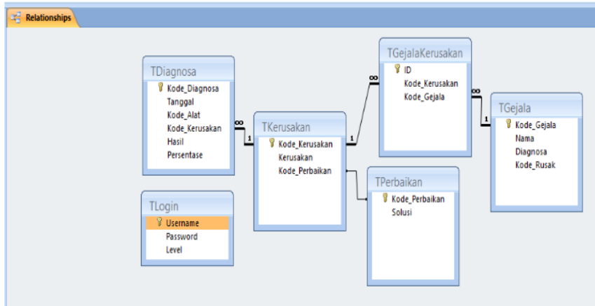
Gambar 2. Relasi tabel
